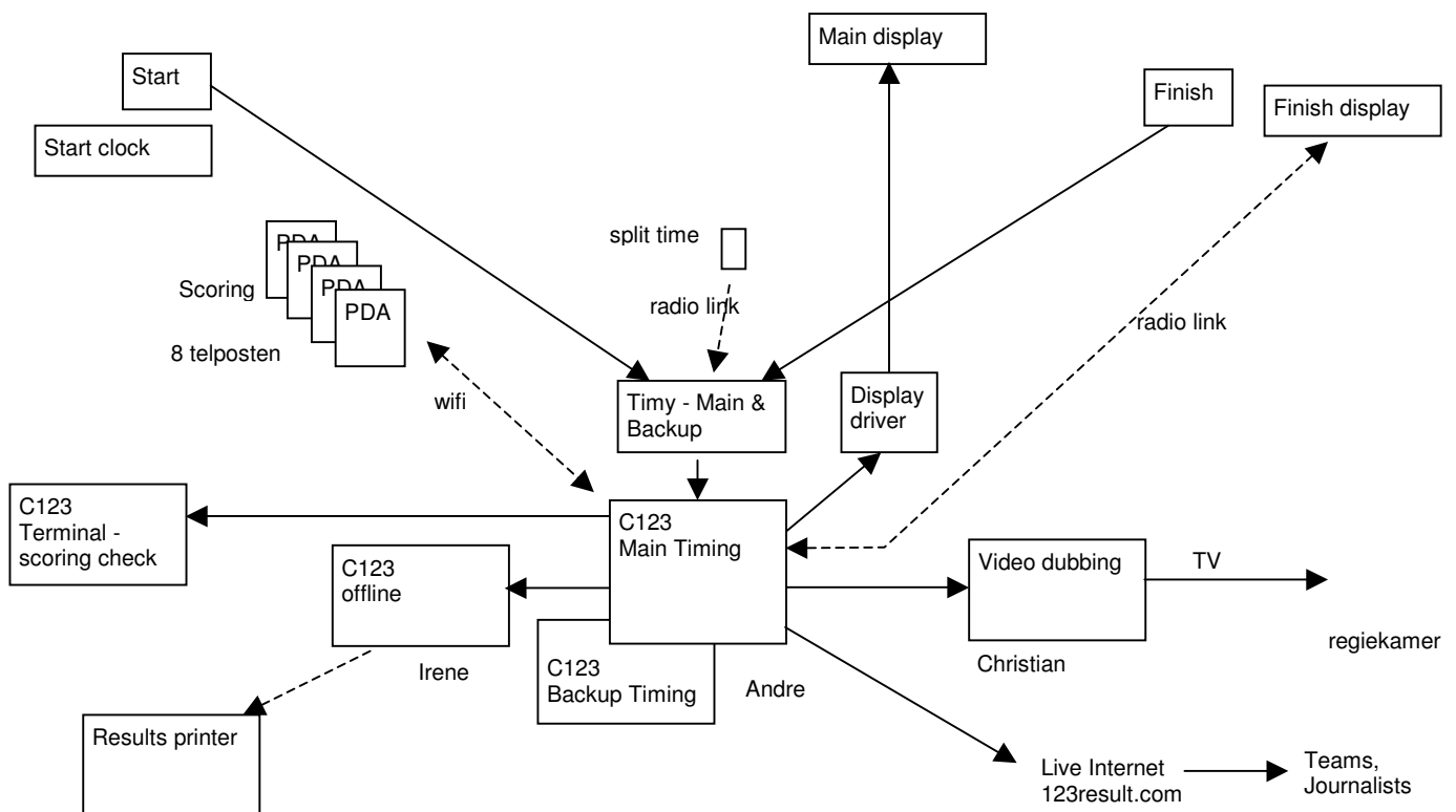
Figuur 1 - Systeemopzet Timing & scoring EK Slalom 2009
