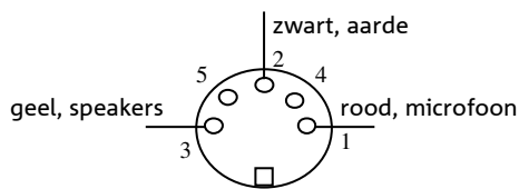
Plug, vooraanzicht
